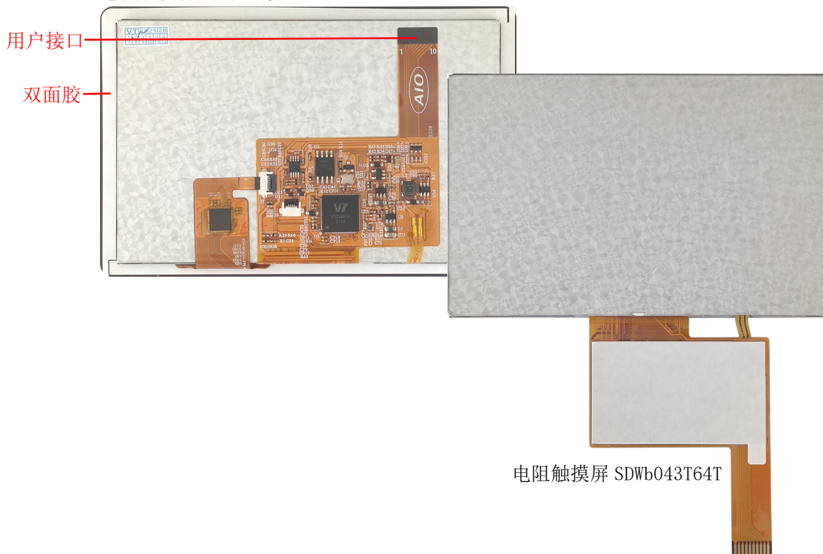
图 1 产品外观及硬件配置图
